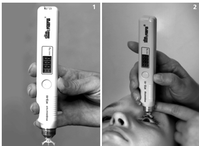
Рисунок 1 Общий вид индикатора ИГД-03 diathera и правильное положение руки исследователя при измерении ВГД
